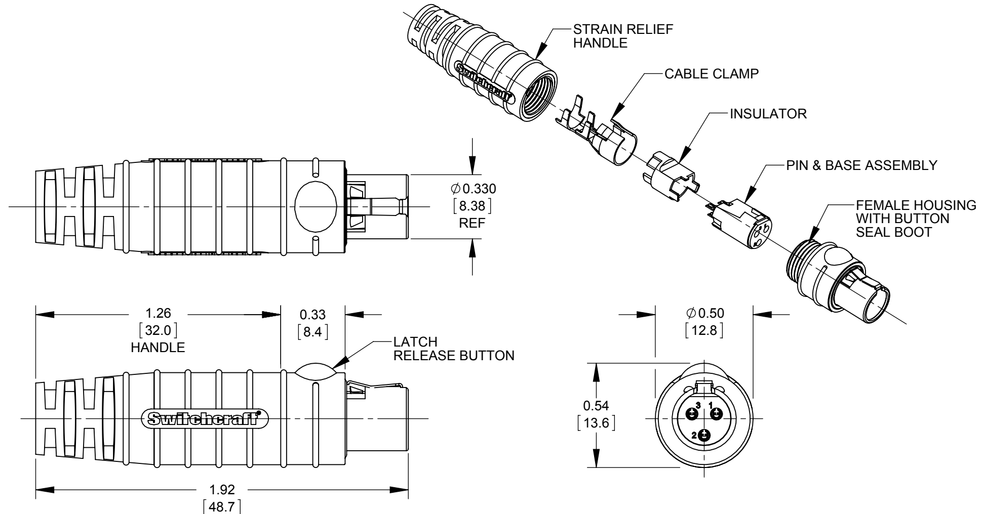
TA3FS SHOWN
